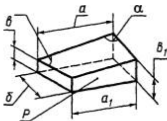
Рисунок 4 - Размеры трапецидального клина с соотношением \frac{v}{a} \leq 1
