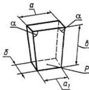
Рисунок 2 - Торцовый клин
