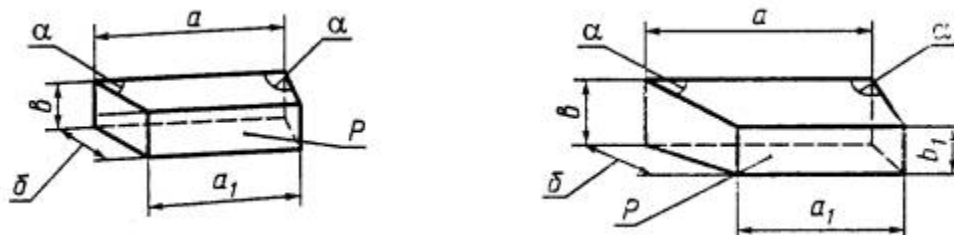
Рисунок 3 - Трапецеидальный клин
